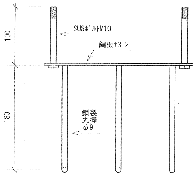
立面図
