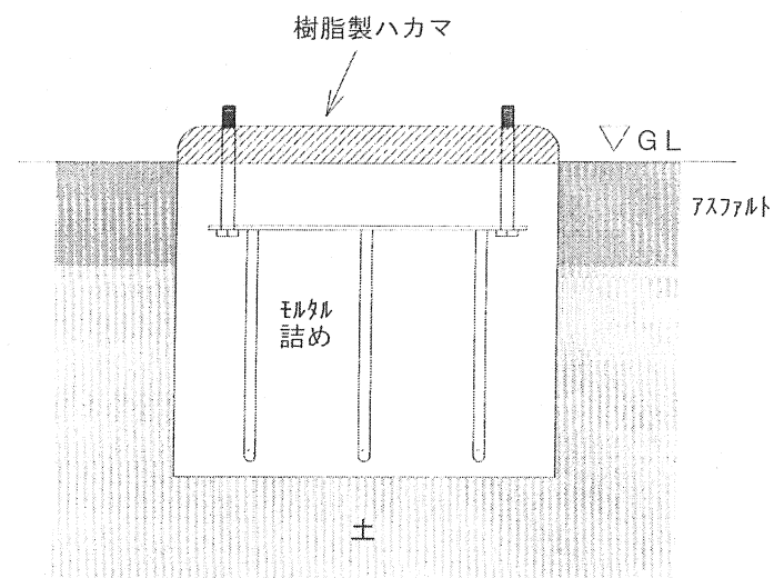
施工図
