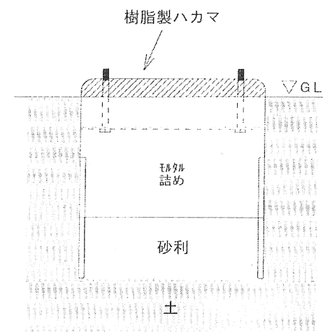
施工図
