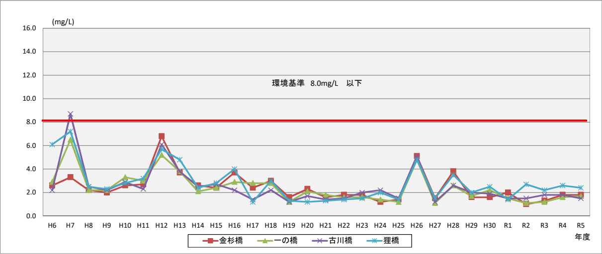
古川のBOD (mg/L)の経年変化(年平均値)
