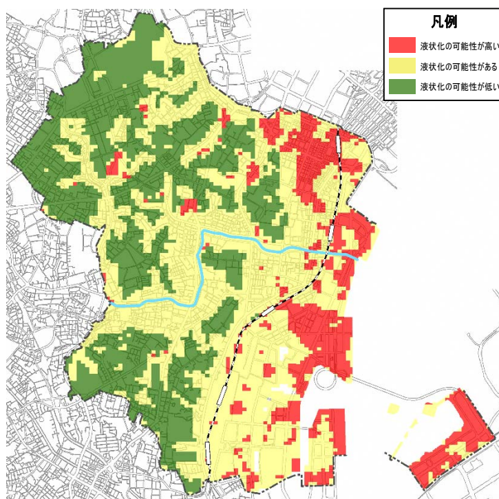
図1-2-15 液状化危険度分布
