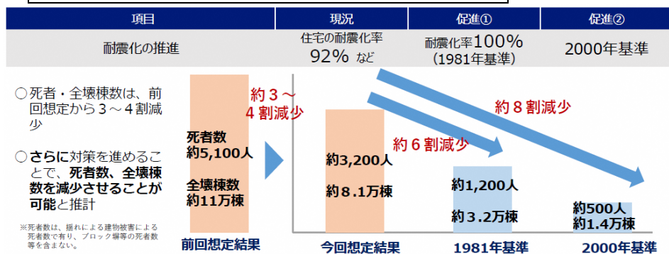
図1-2-5 耐震化率の向上による被害軽減効果
