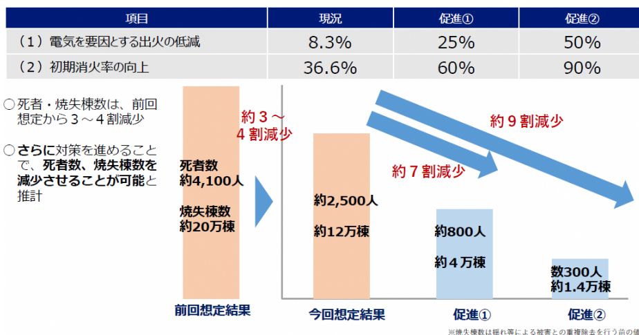
図1-2-7 出火抑制対策による被害軽減効果
