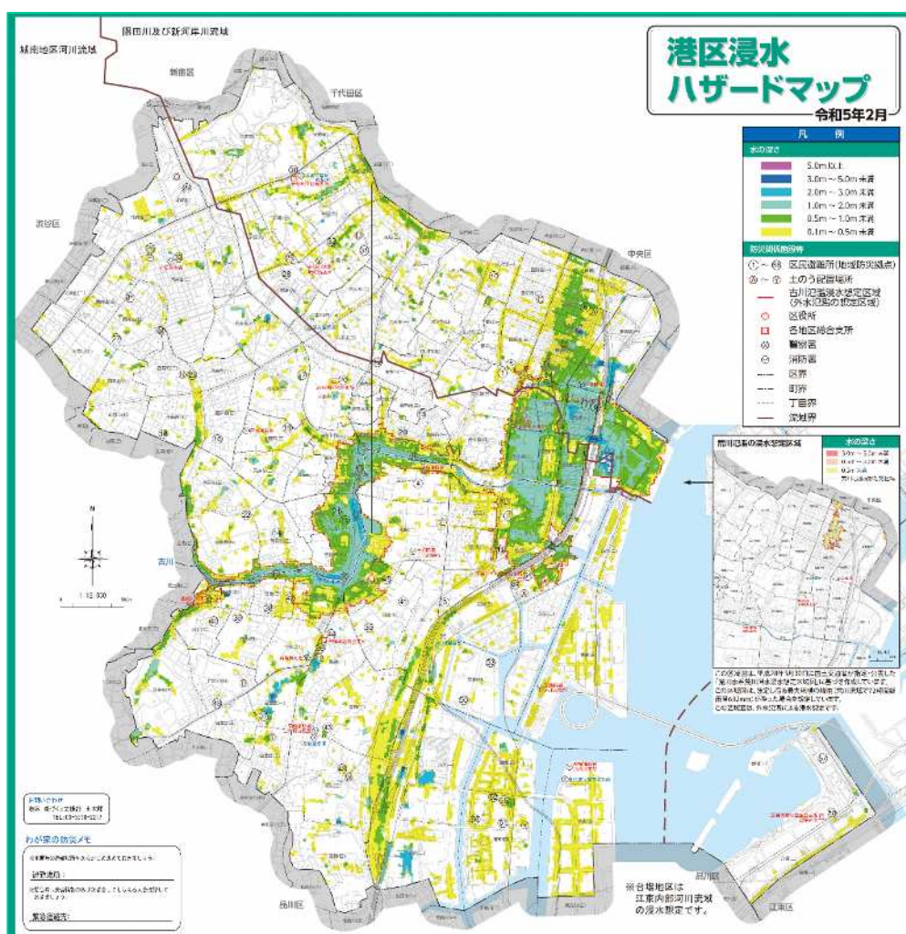
図1-2-9 港区内の浸水予想区域図
