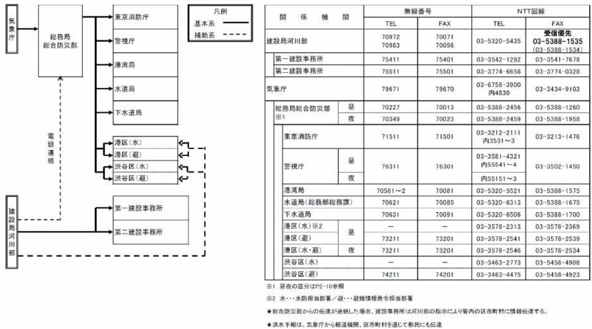
図3-5-4 渋谷川・古川洪水予報伝達系統図
