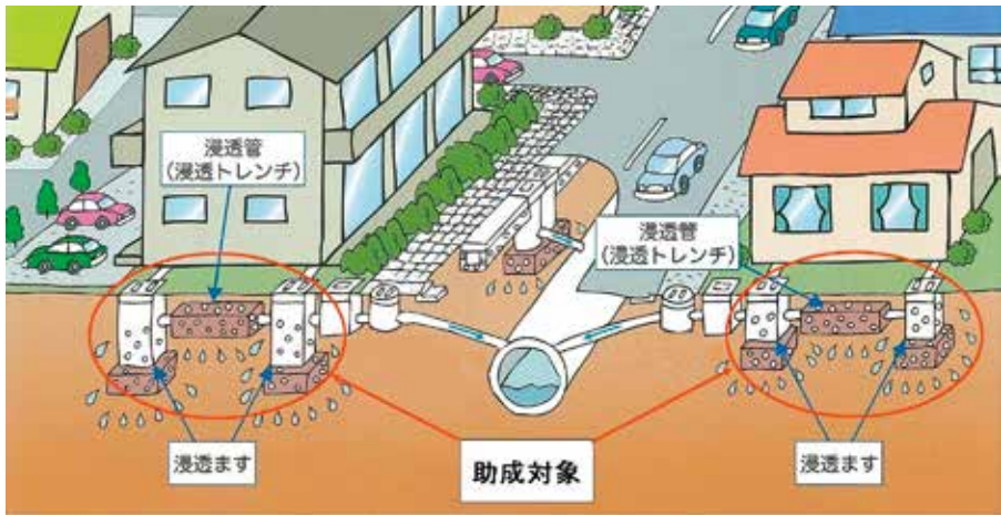
雨水浸透施設設置のイメージ図
