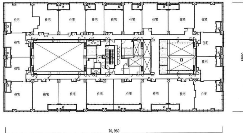
34階平面図
