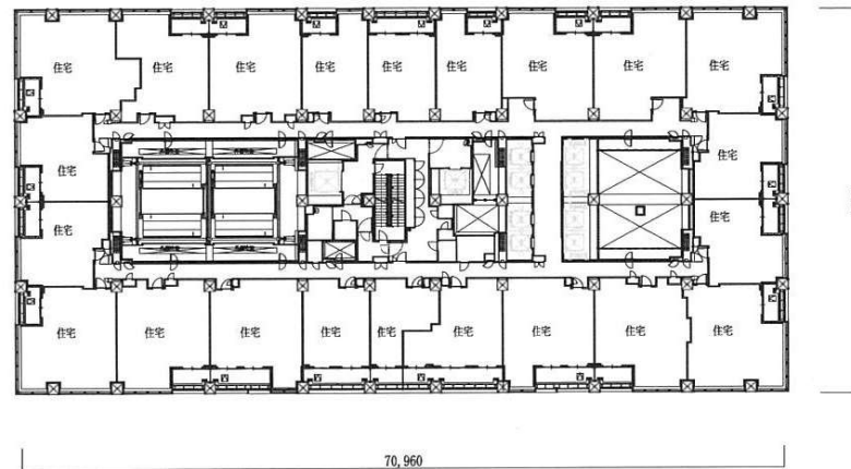
26階平面図
