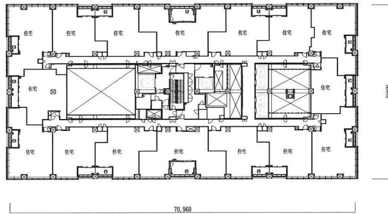
43階平面図
