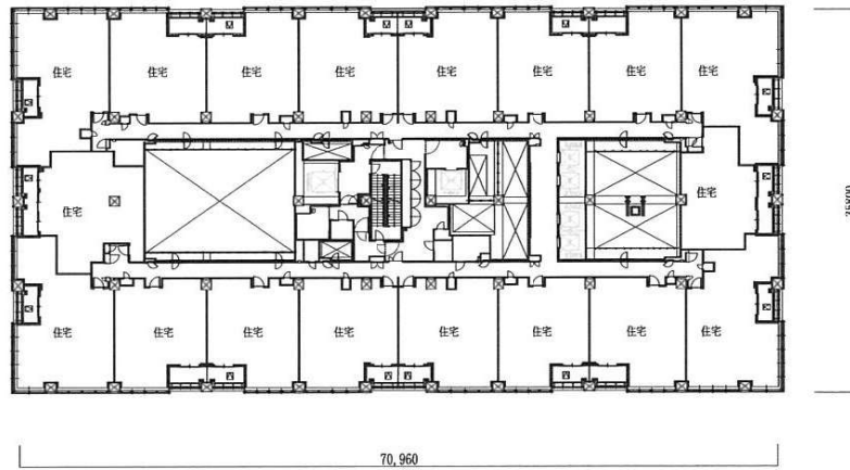
39階平面図
