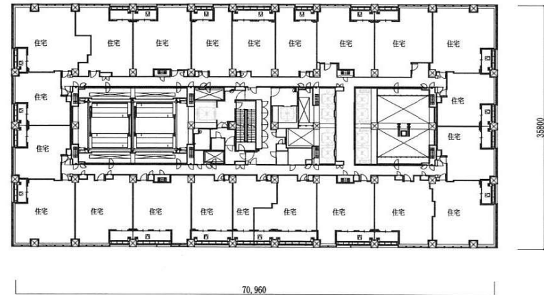
25階平面図
