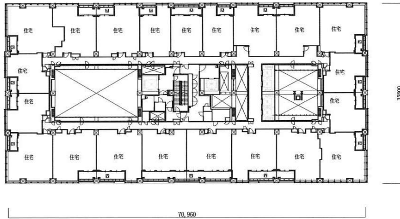
35階平面図
