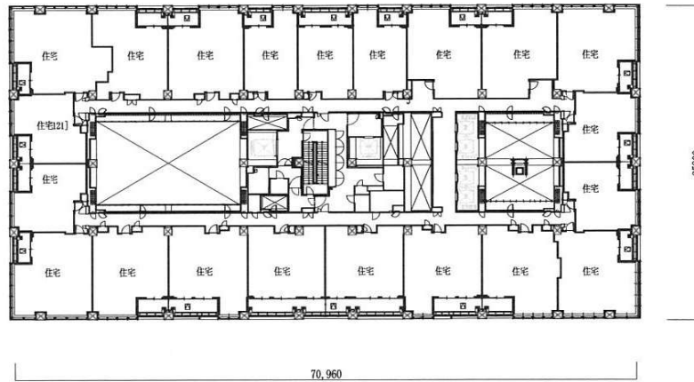
31階平面図
