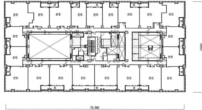
33階平面図
