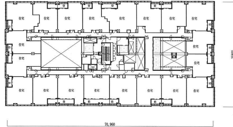
37階平面図
