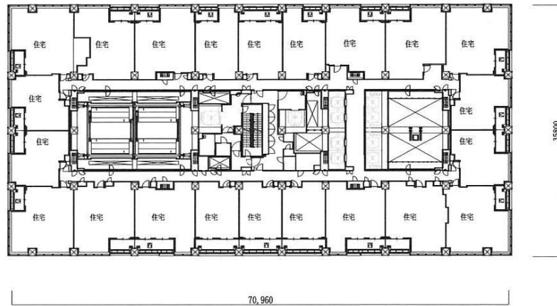
23階平面図
