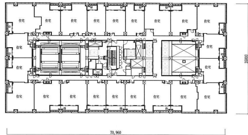
24階平面図
