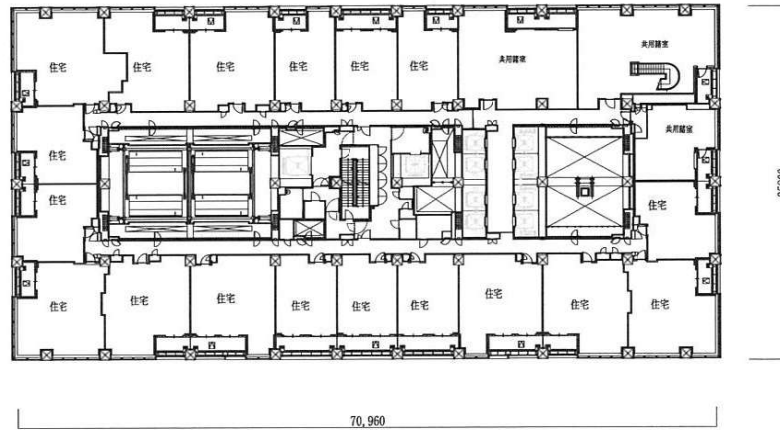
(EV乗継階) 27階平面図
