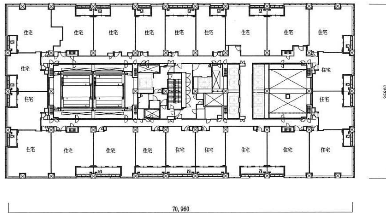
22階平面図
