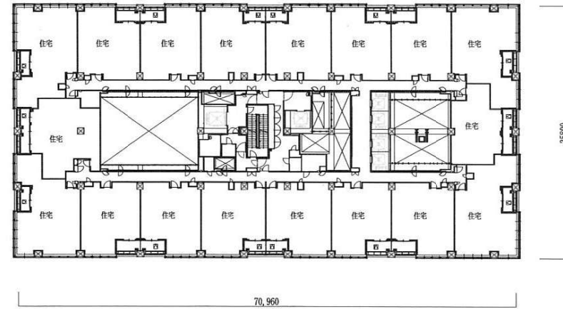
41階平面図
