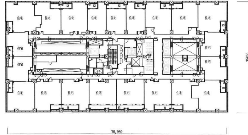
29階平面図
