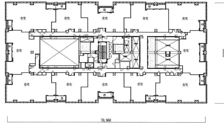
45階平面図
