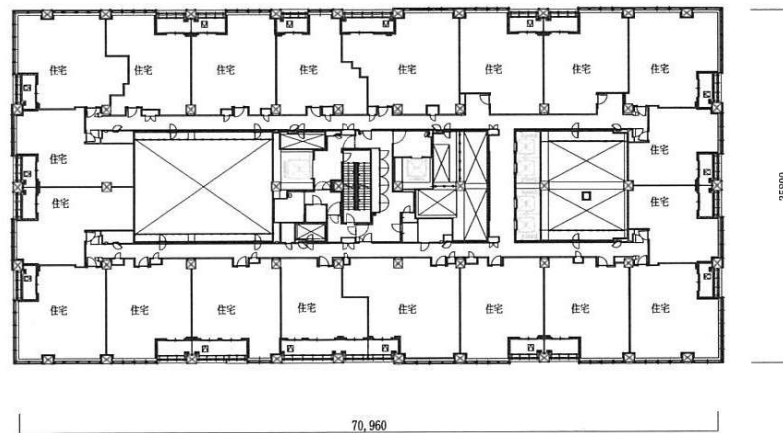
38階平面図
