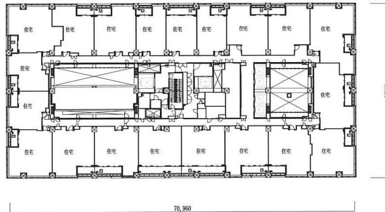
30階平面図
