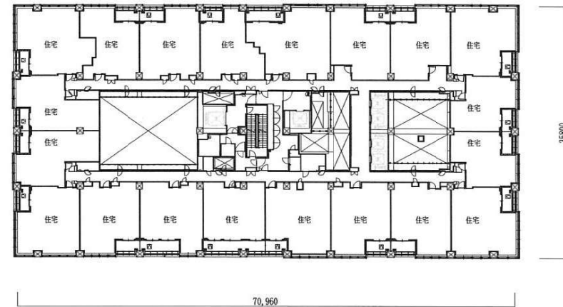
36階平面図
