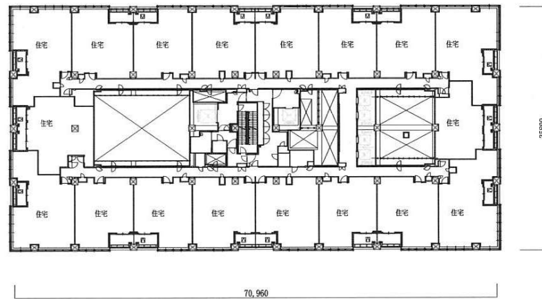
42階平面図
