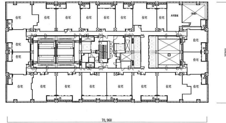
28階平面図
