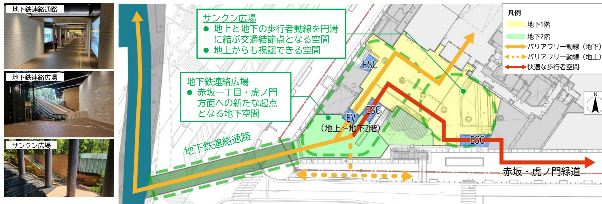
図表2.5-2 溜池山王駅直結の地下鉄連絡通路・地下鉄連絡広場の整備
