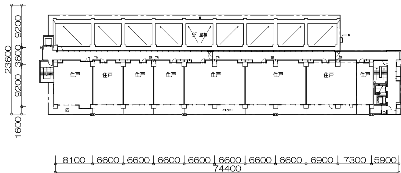
9階平面図
