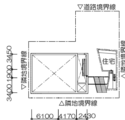
3階平面図
