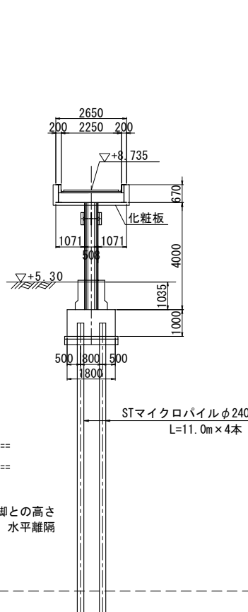
P5橋脚断面図 S=1:200
