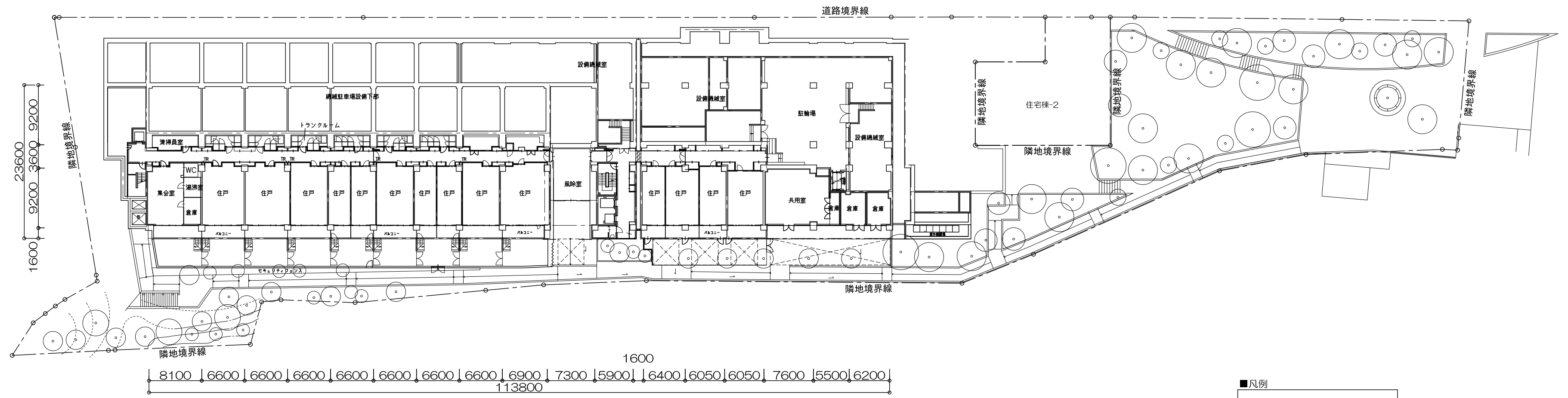
B1階平面図
