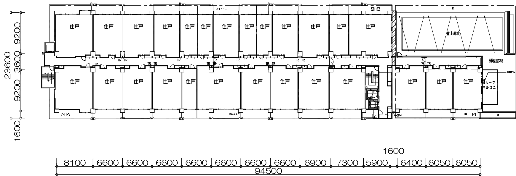
6階平面図
