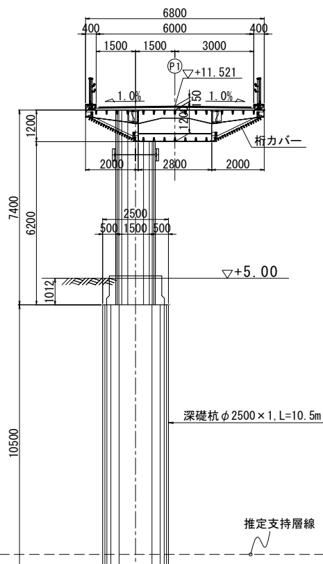
P1橋脚断面図 S=1:200
