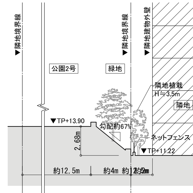
D-D断面図 S=1:200
