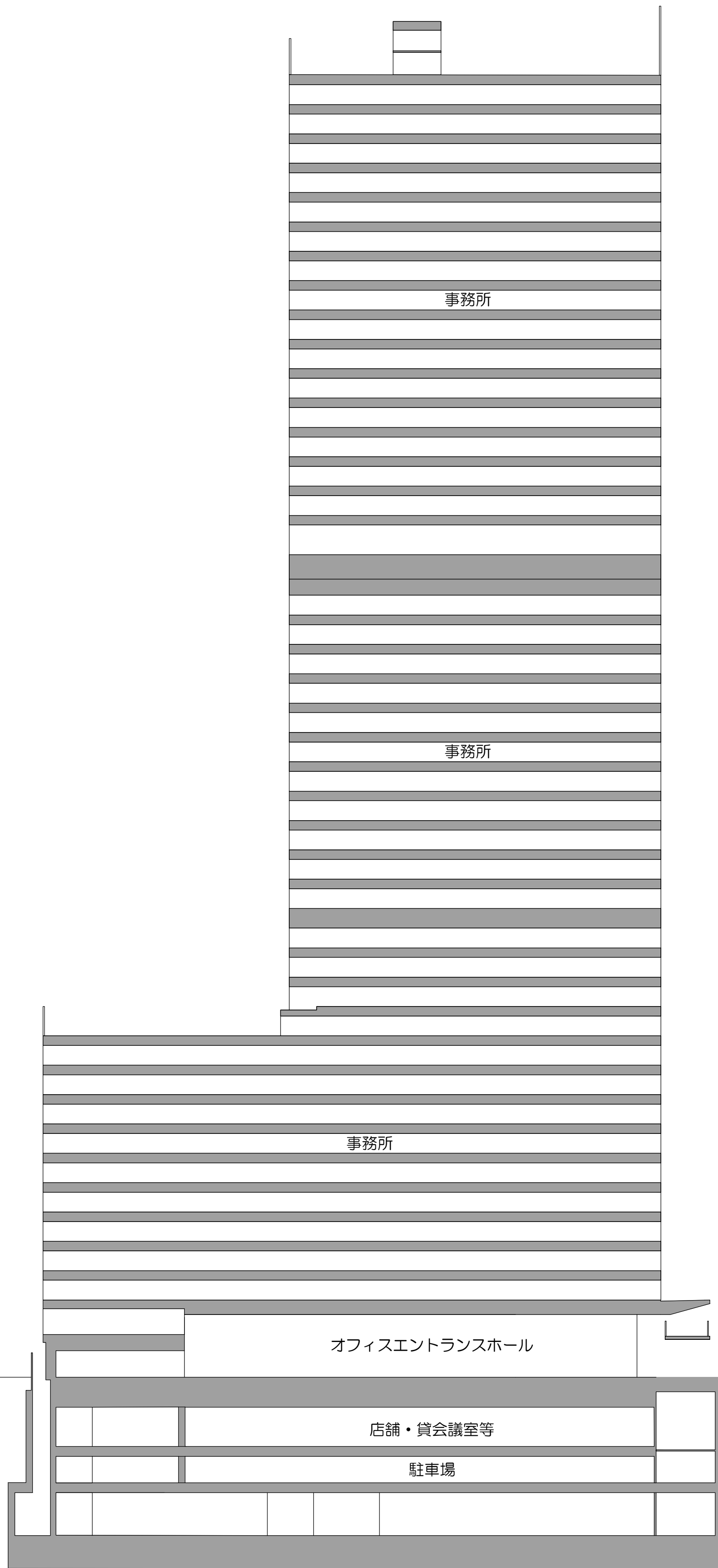
A-A断面図
