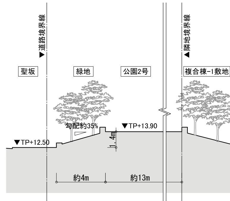
C-C断面図 S=1:200
