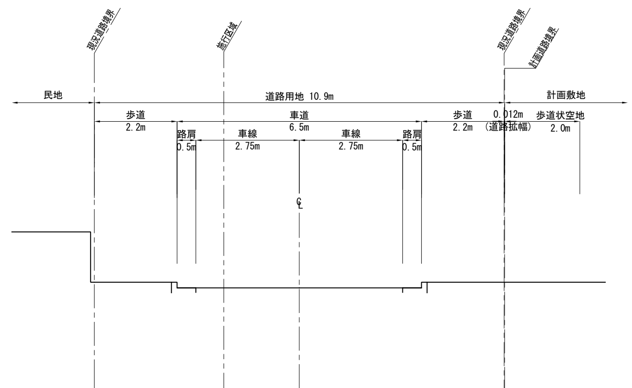
C - C 断面
