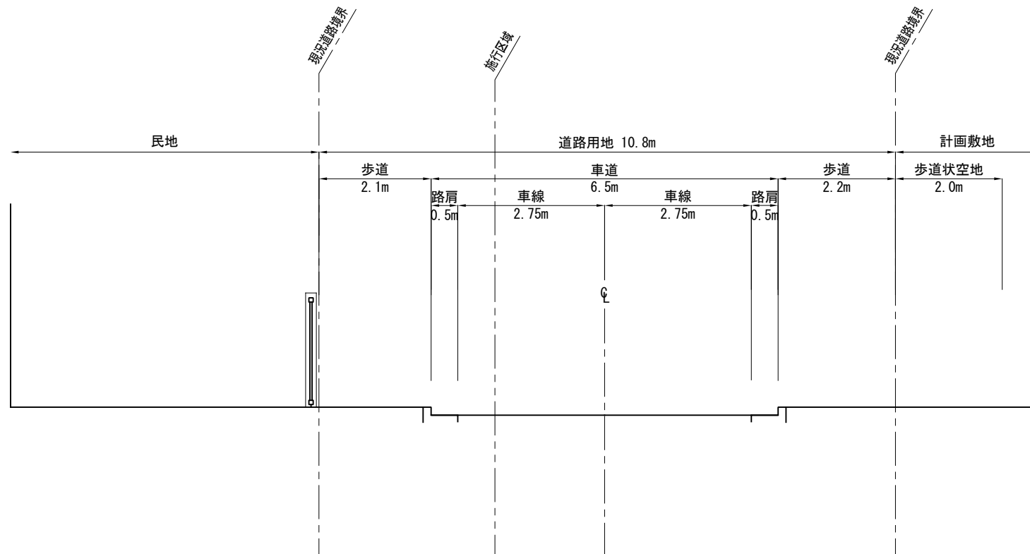
B - B 断面
