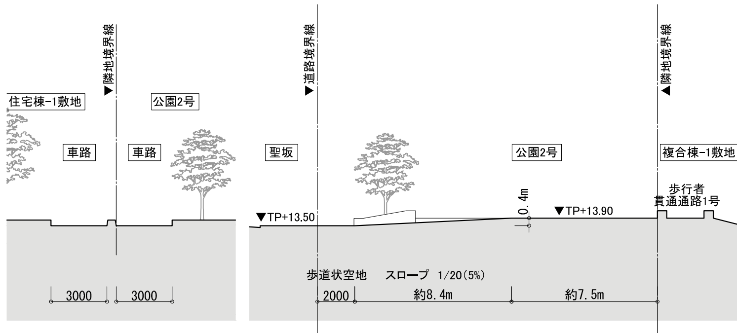
A-A断面図 S=1:200
