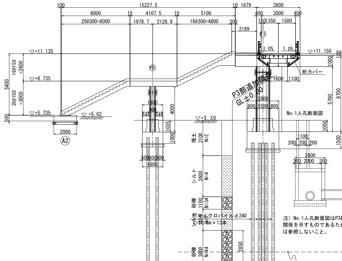
P3橋脚断面図 S=1:200
