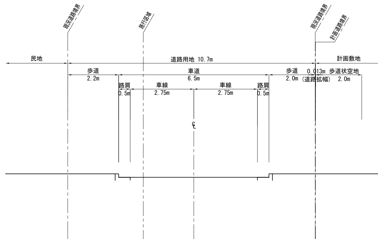
A - A 断面
