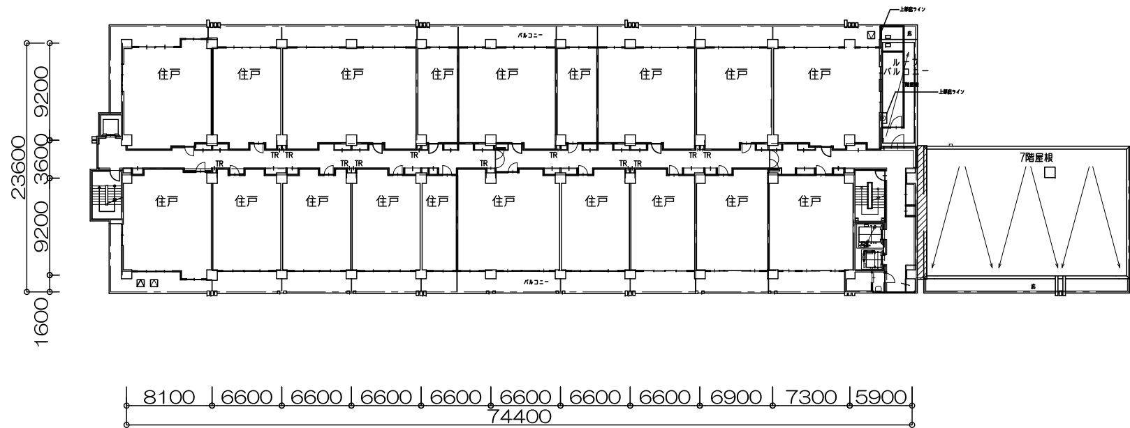
7階平面図
