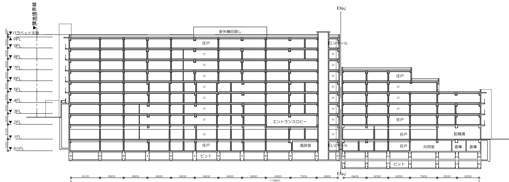
B-B断面図
