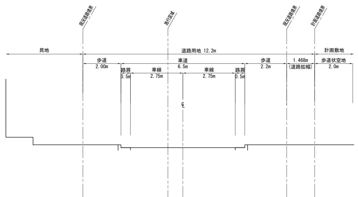
D - D 断面
