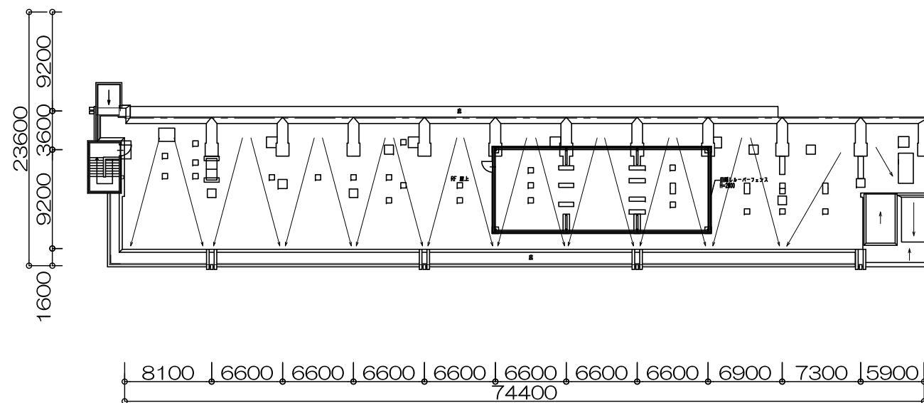
屋上階平面図
