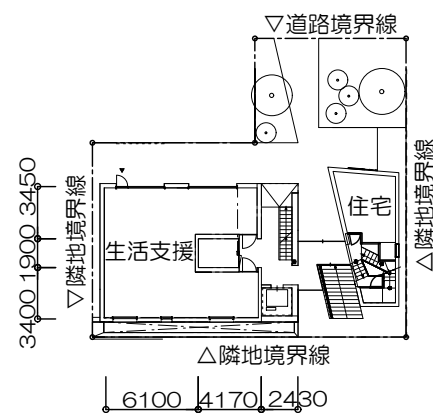
1階平面図
