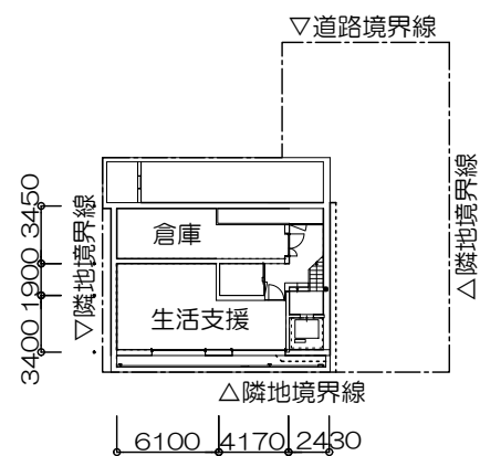
地下2階平面図
