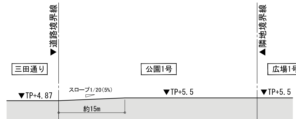
B-B断面図
