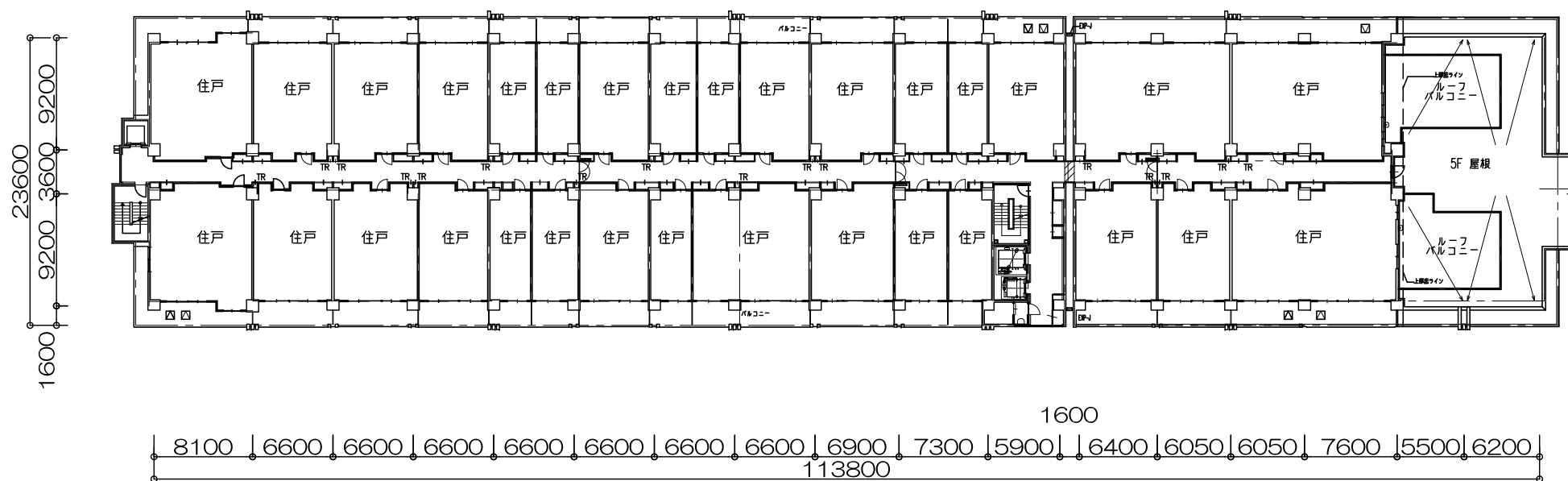
5階平面図
