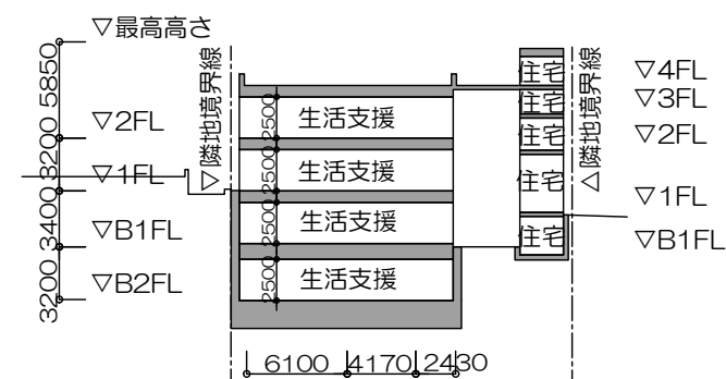
B-B断面図
