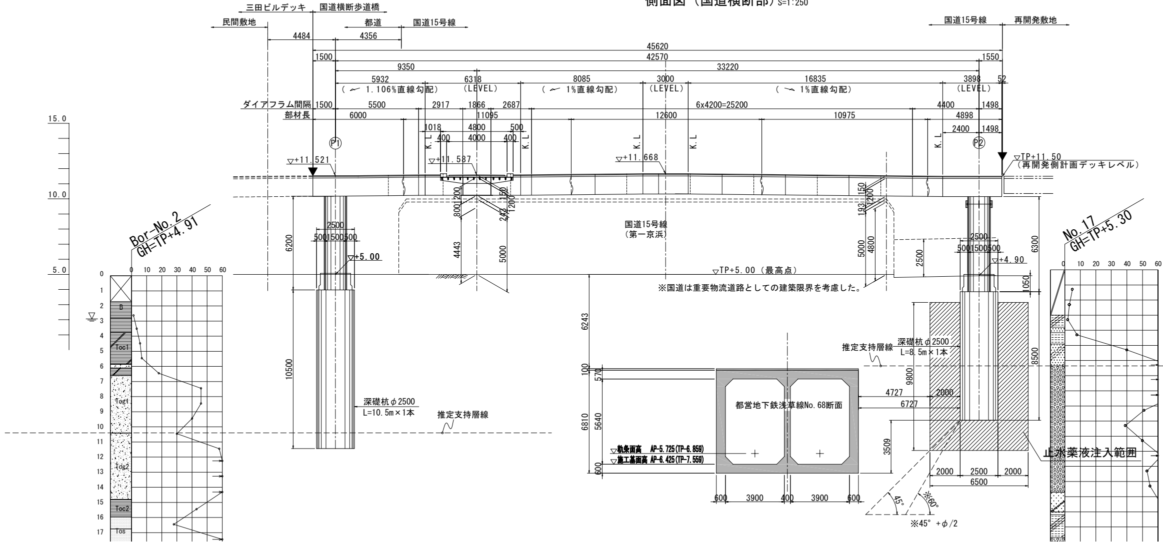
P1橋脚断面図 S=1:200
