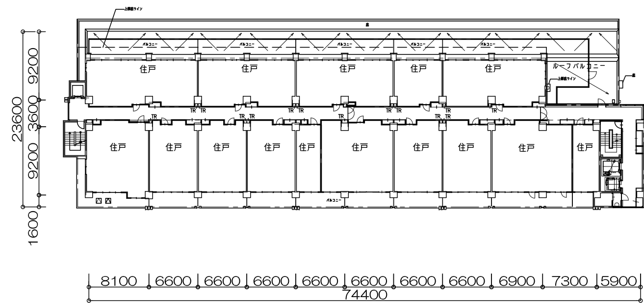
8階平面図
