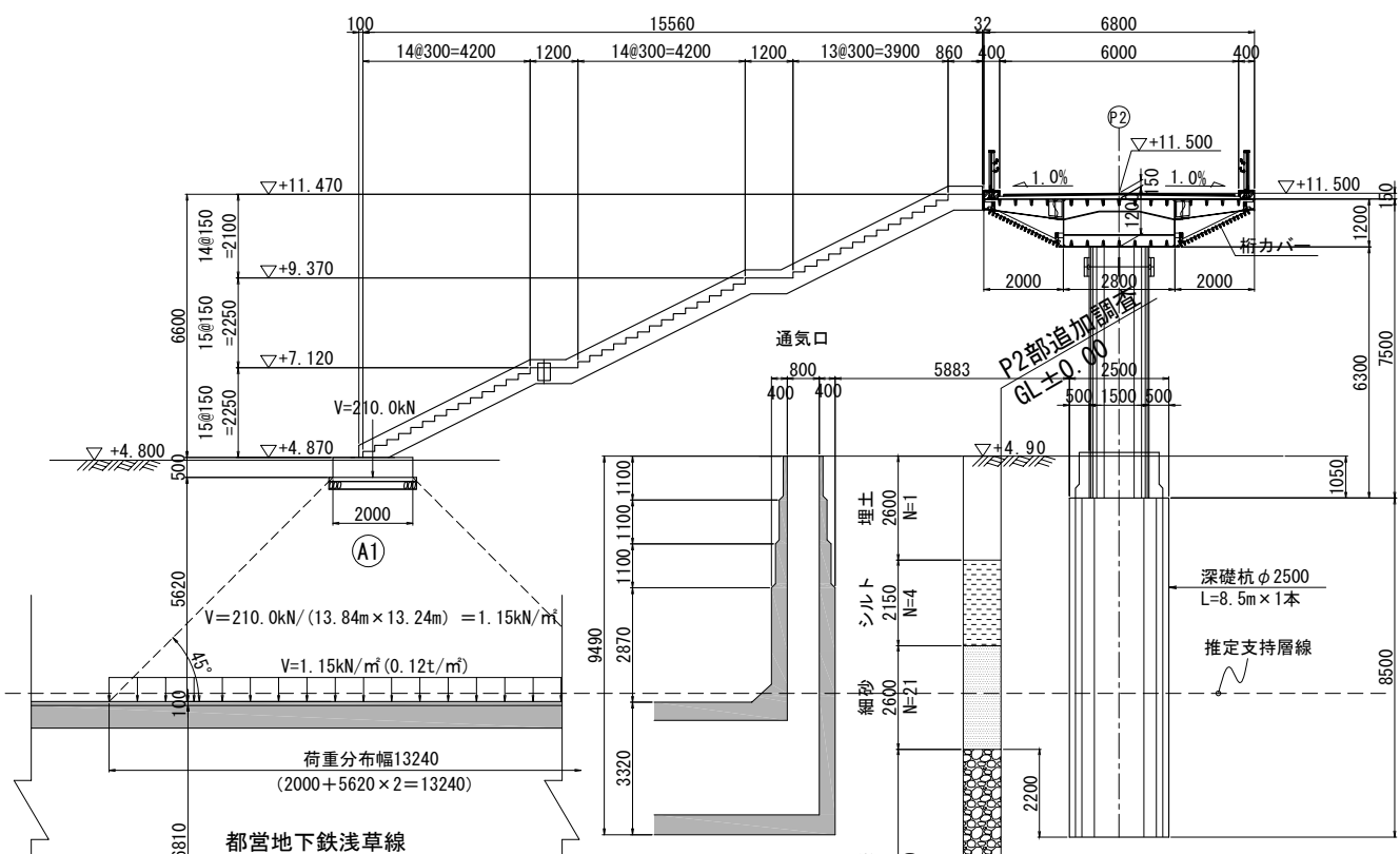
P2橋脚断面図 S=1:200
