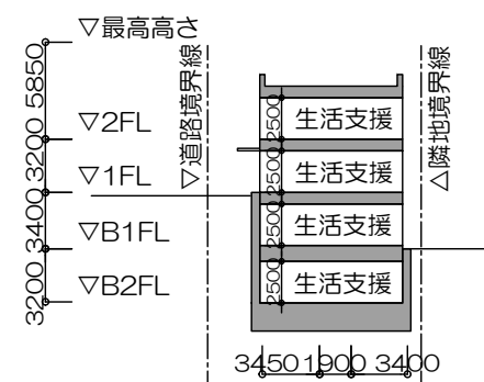
A-A断面図
