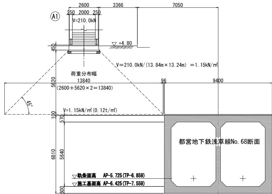
A1橋台断面図 S=1:200
