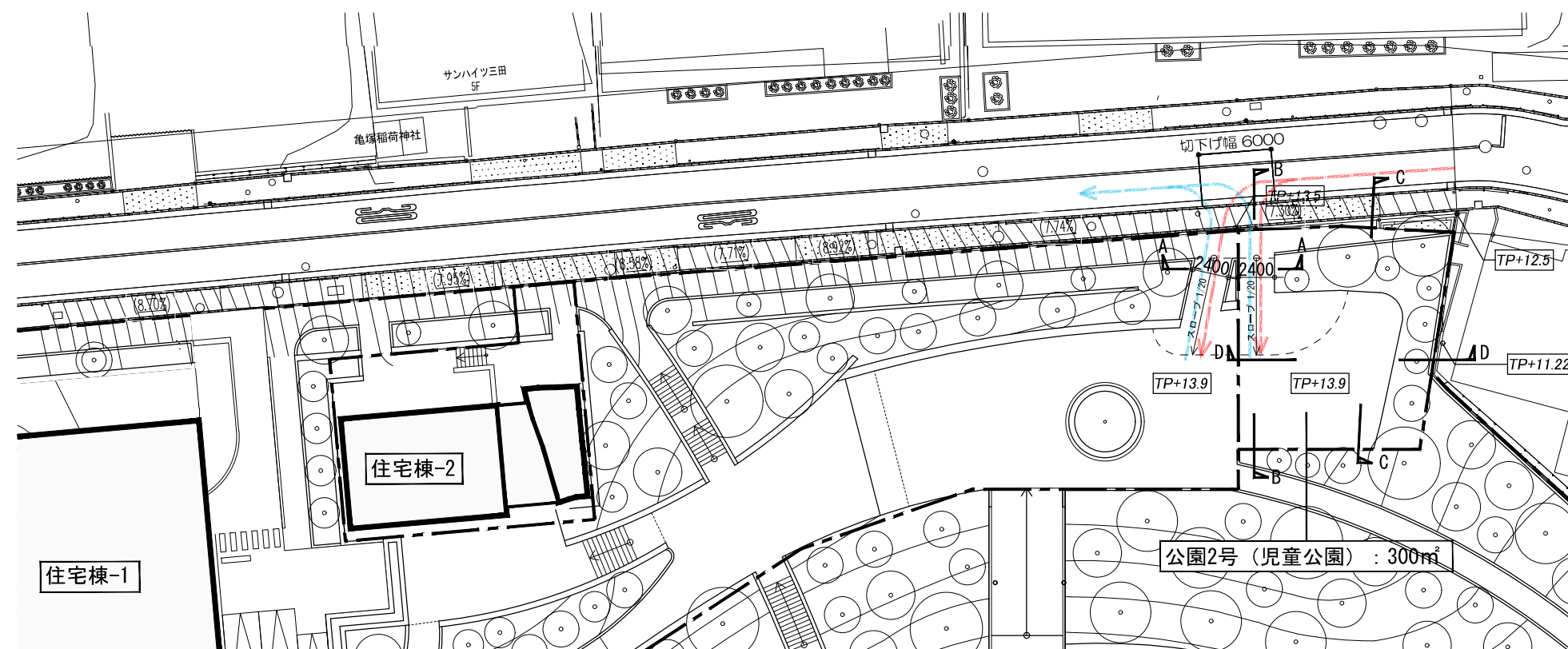
公園2号平面図 S=1:500
