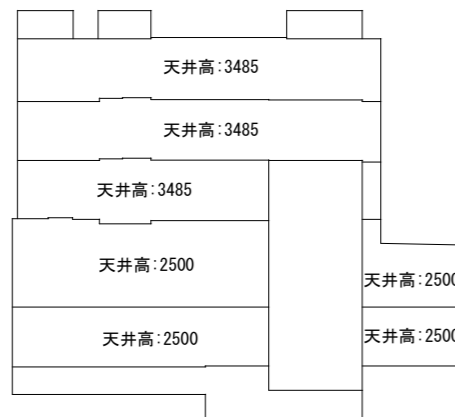
d-d' 断面図
