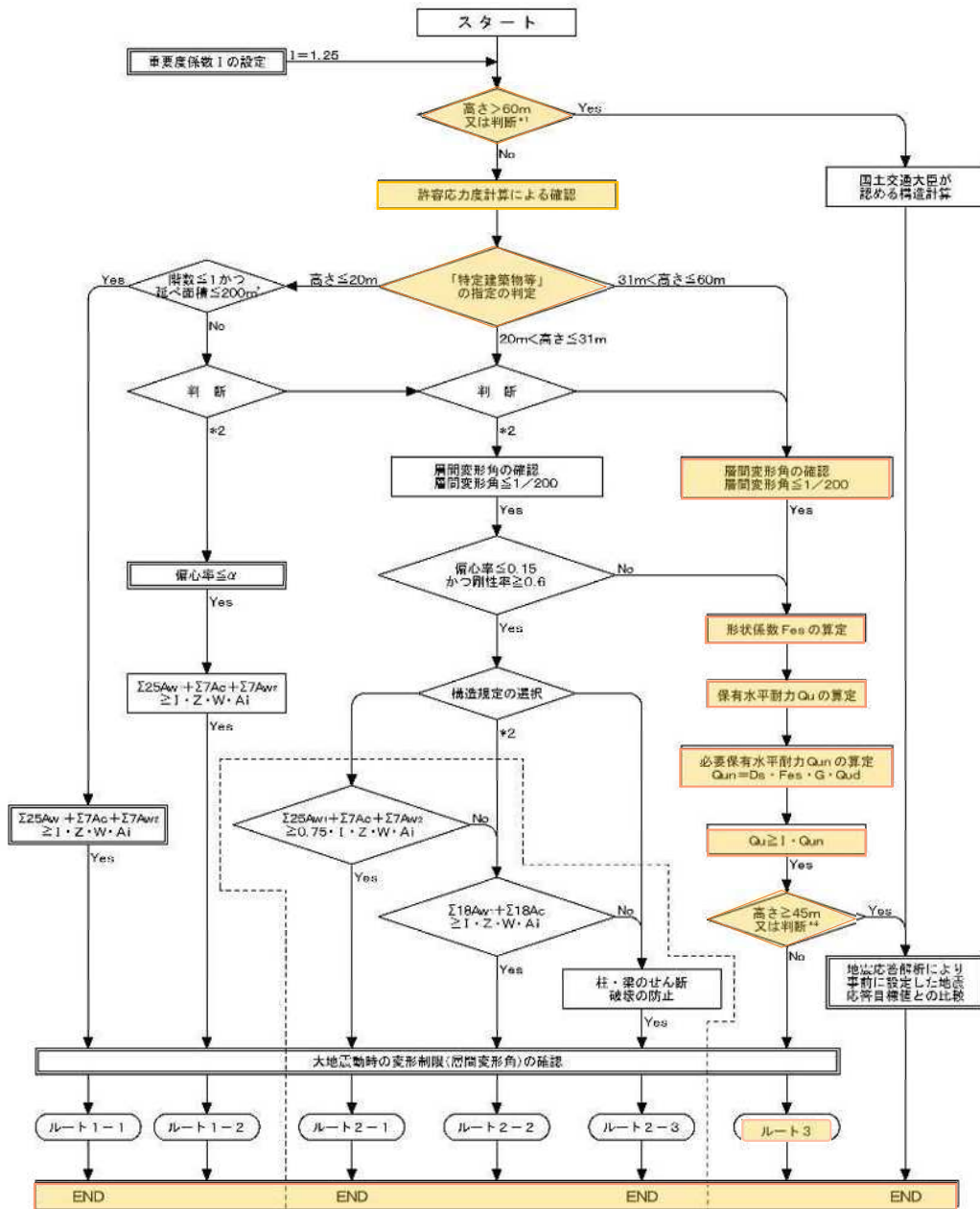
鉄筋コンクリート造の構造計算フロー
