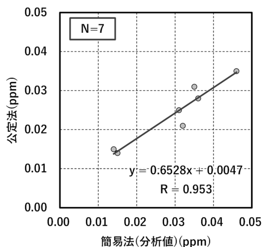
図2-1 二酸化窒素(NO 2 )の簡易法(分析値)と公定法の回帰式(地点D 7 )
