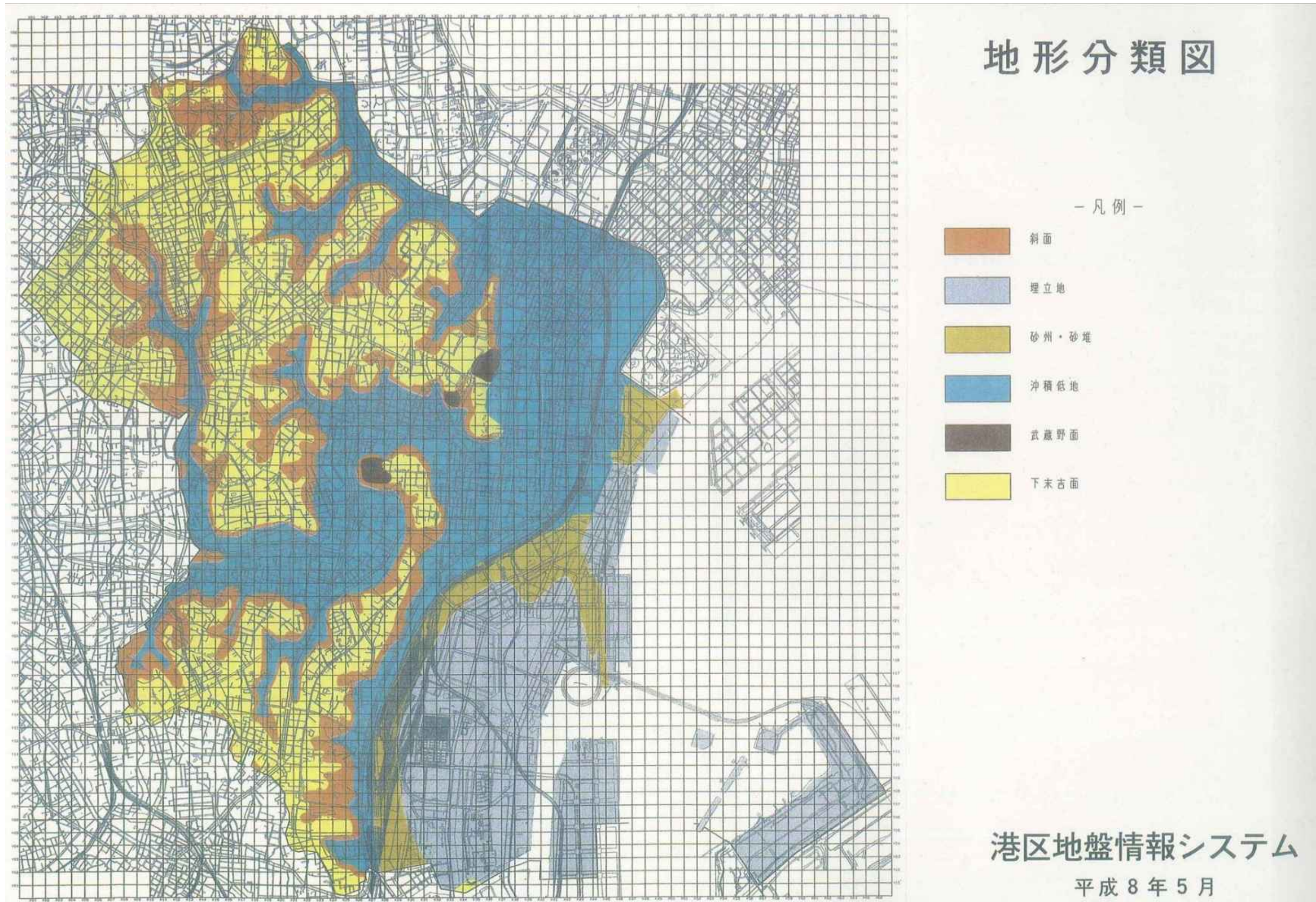
震1-2-1 地形分類図
