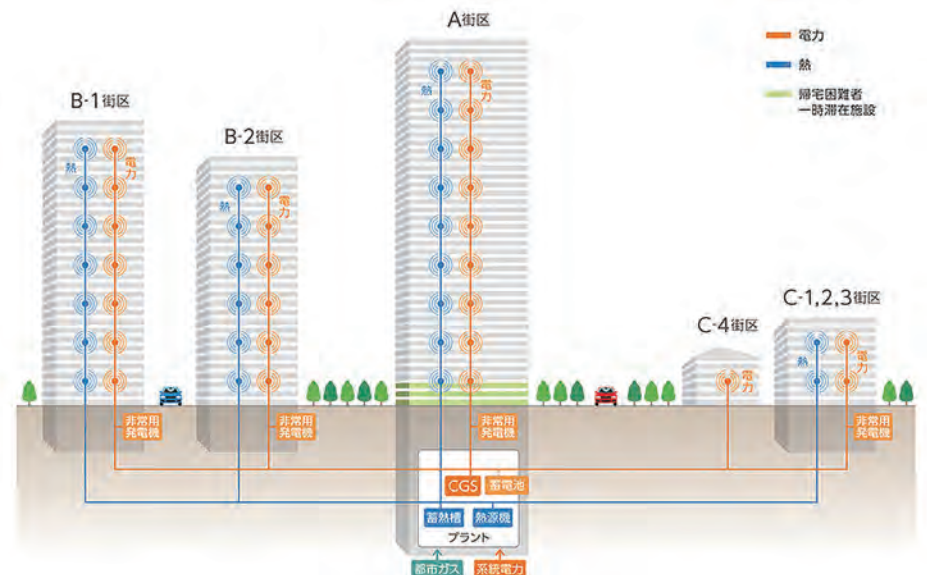
【図2】麻布台ヒルズのエネルギー供給の仕組み
