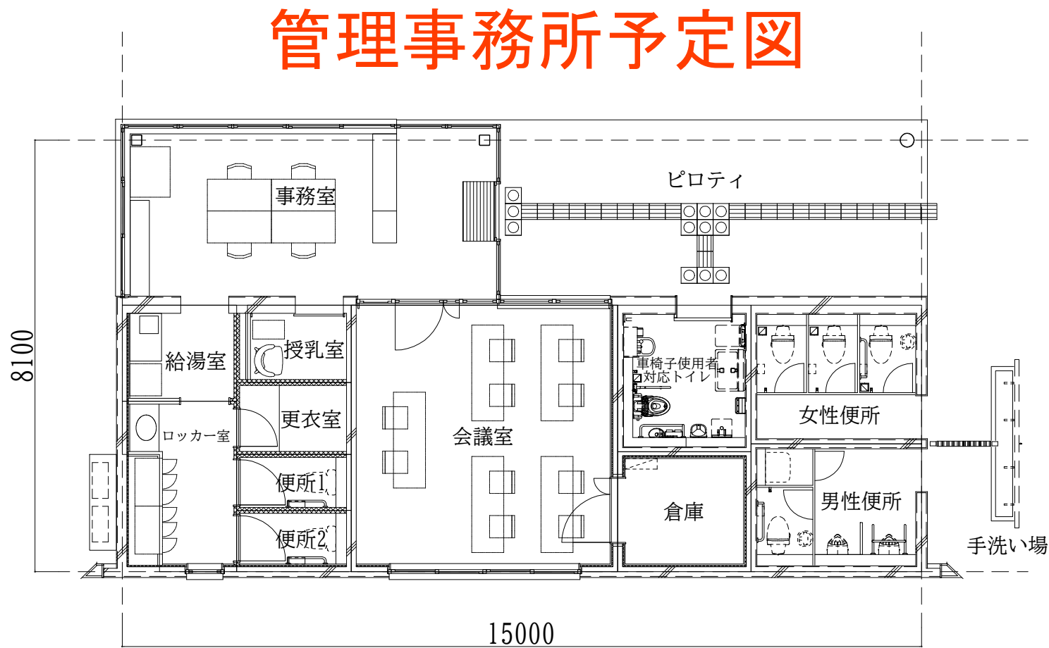
地上1階平面図 縮尺1／500
