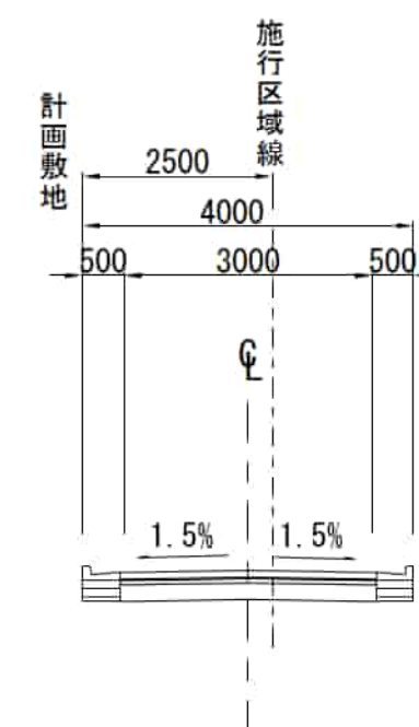
特別区道第1191号線 (区画道路4号) (F-F')
