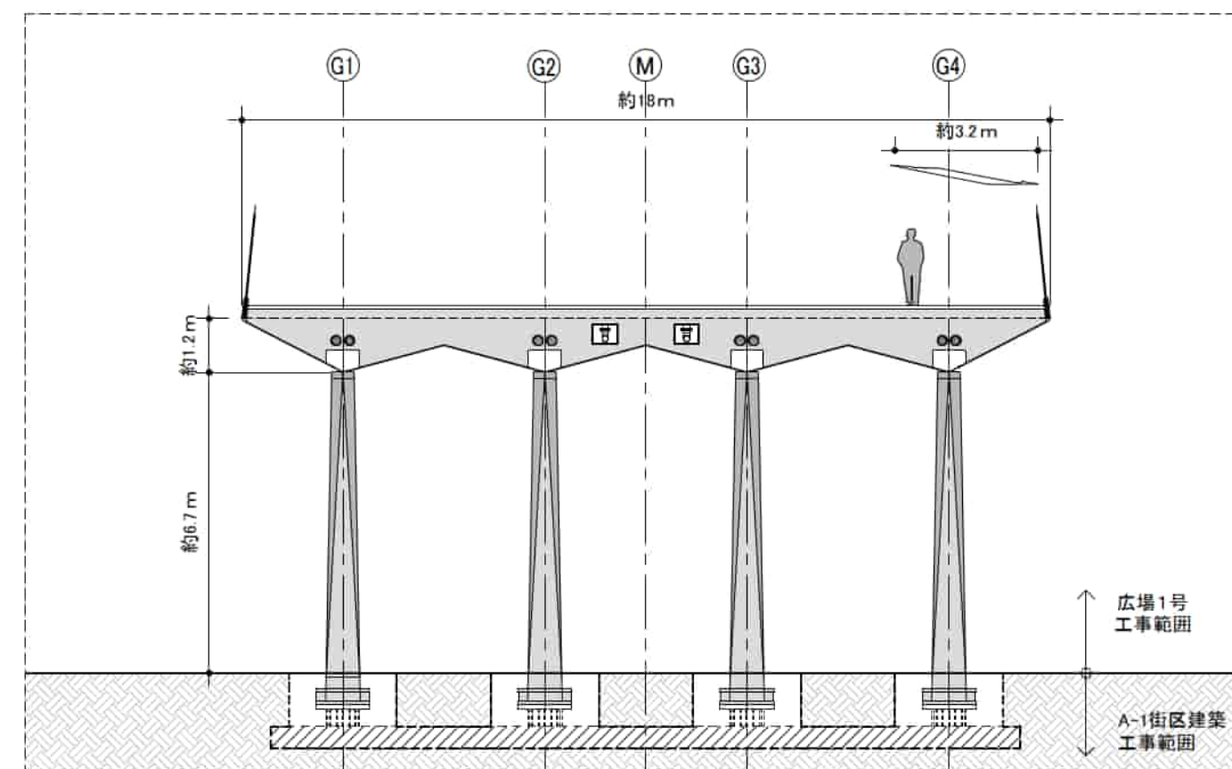
断面図C-C'
