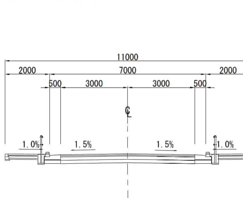
特別区道第128号線 (区画道路2号) (E-E')
