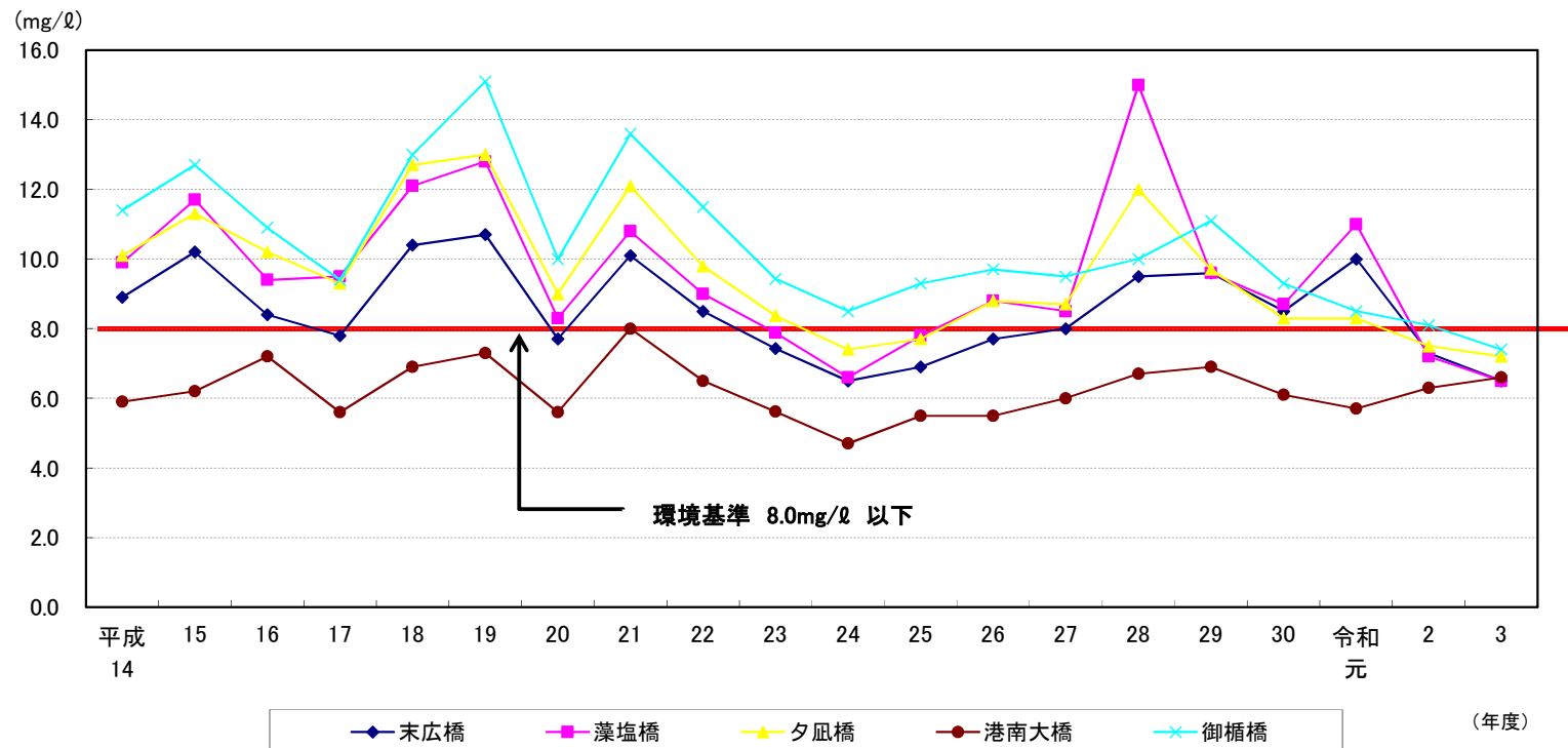
運河のCOD (mg/L) の経年変化 (年平均値)
