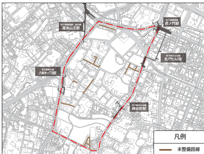
電線類地中化の未整備路線 (電線類地中化推進計画(素案)(令和4(2022)年2月)を基に作成)
