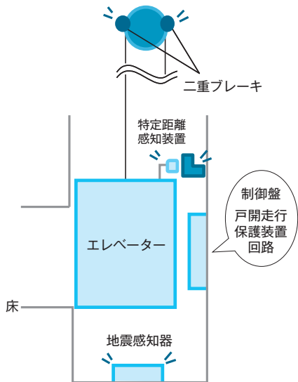
図1 エレベーター概要図(横から見た図)
