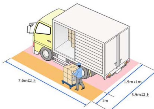
図 9 荷捌き車の駐車施設の車室の大きさ
