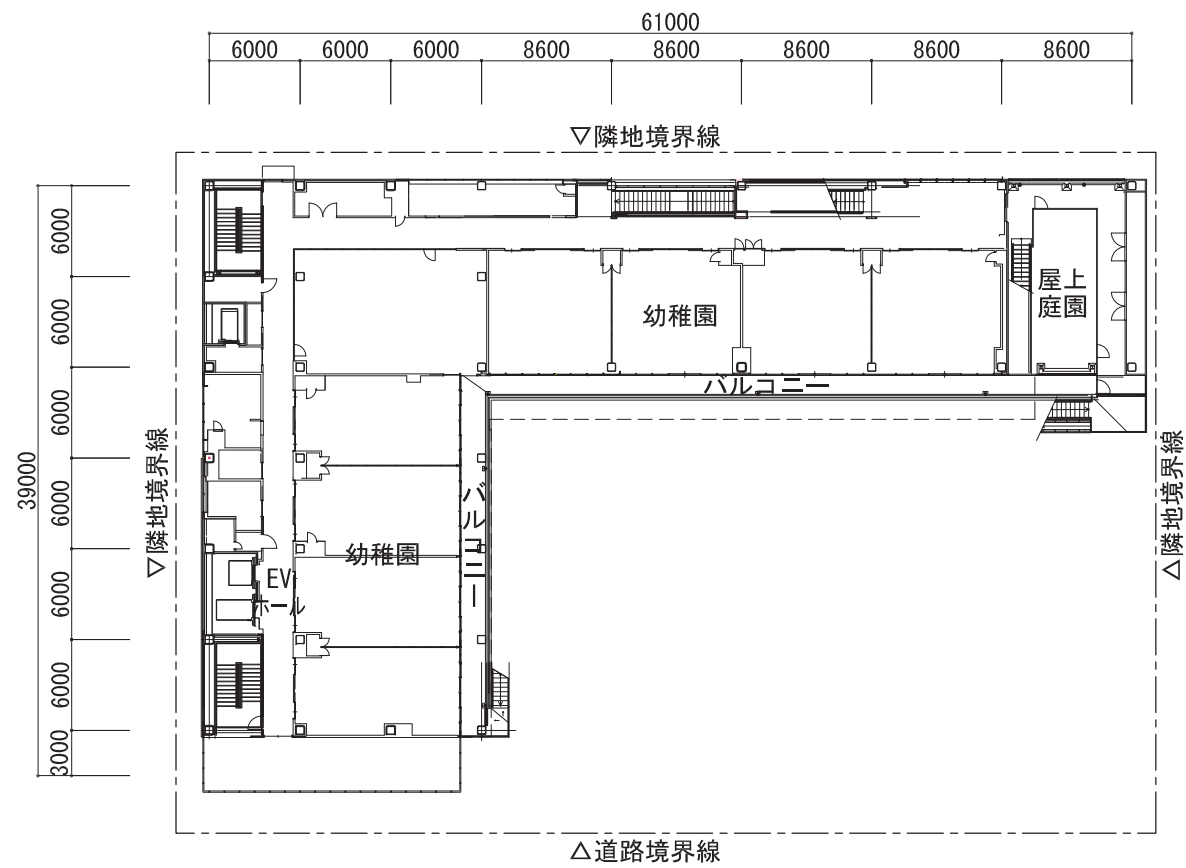
2階平面図
