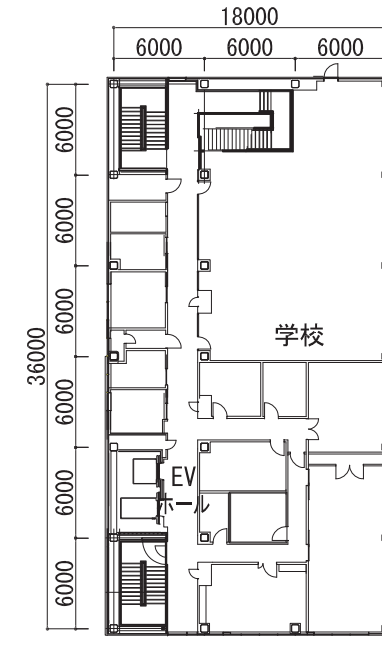
6階平面図
