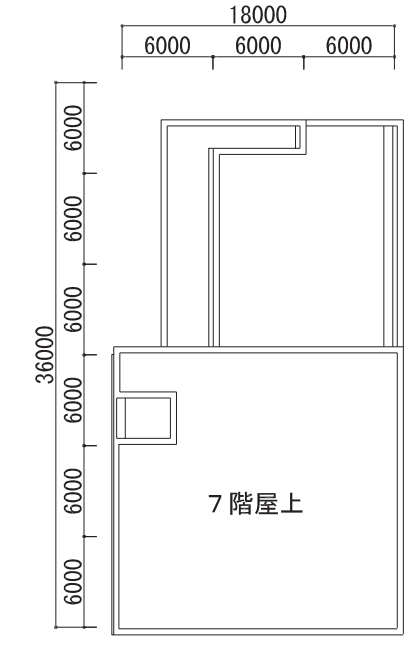
屋上平面図
