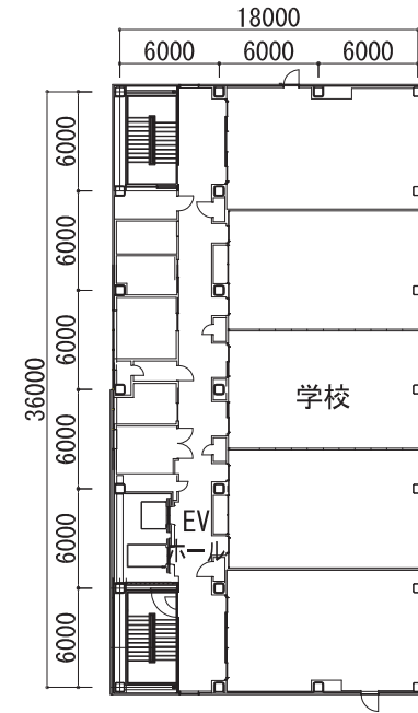
5階平面図
