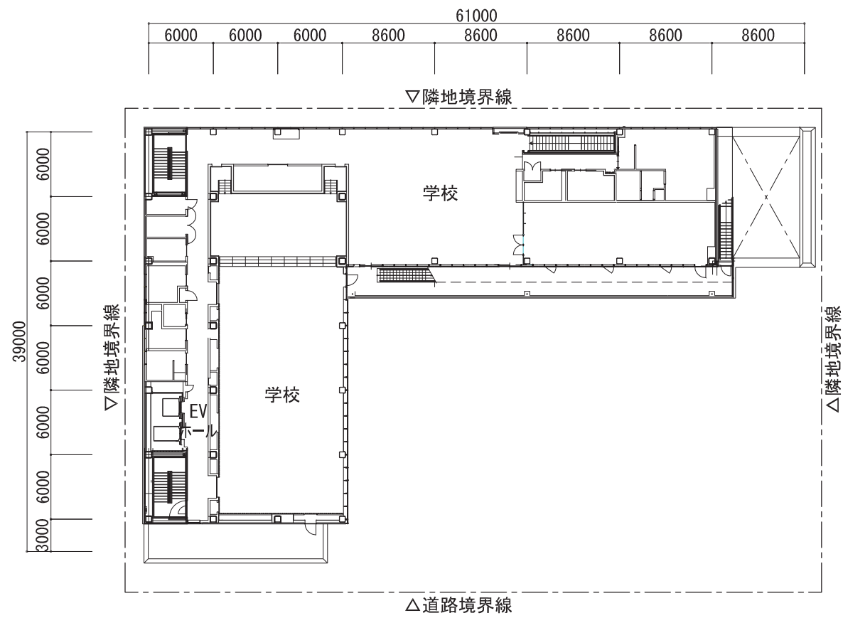
3階平面図
