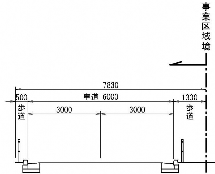
A-A 断面
