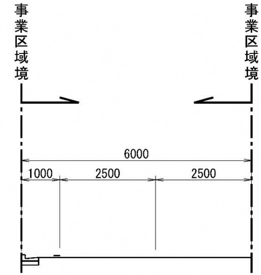
D-D 断面
