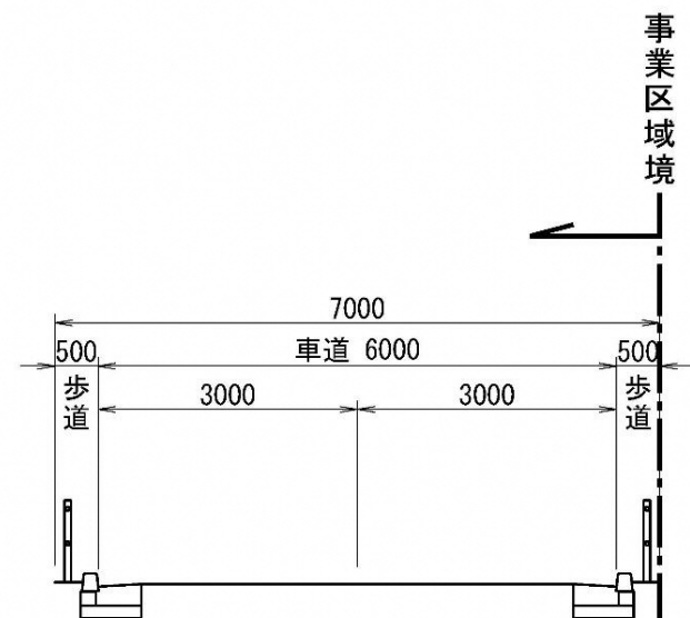
B-B 断面
