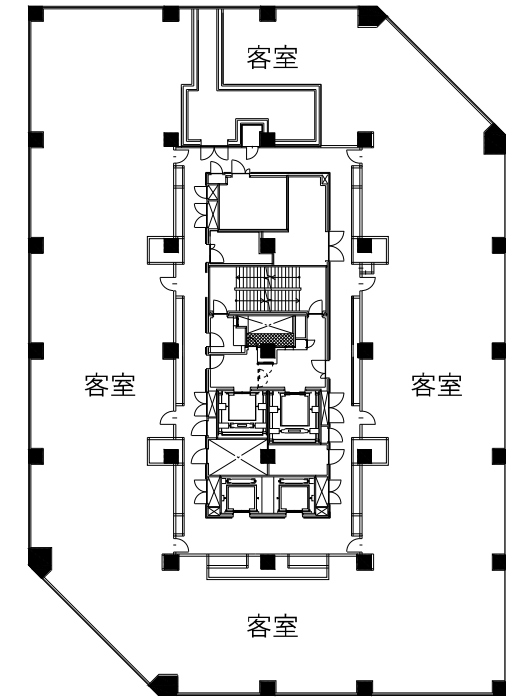
48階平面図 S=1/250(A1),S=1/500(A3)
