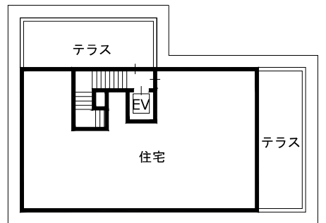
3階平面図
