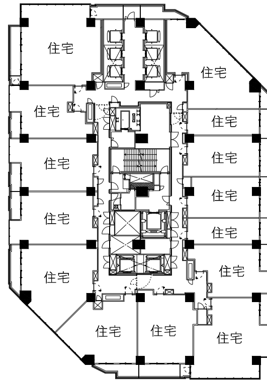
15~21階平面図 S=1/250(A1),S=1/500(A3)
