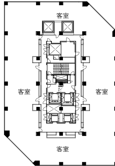
47階平面図 S=1/250(A1),S=1/500(A3)
