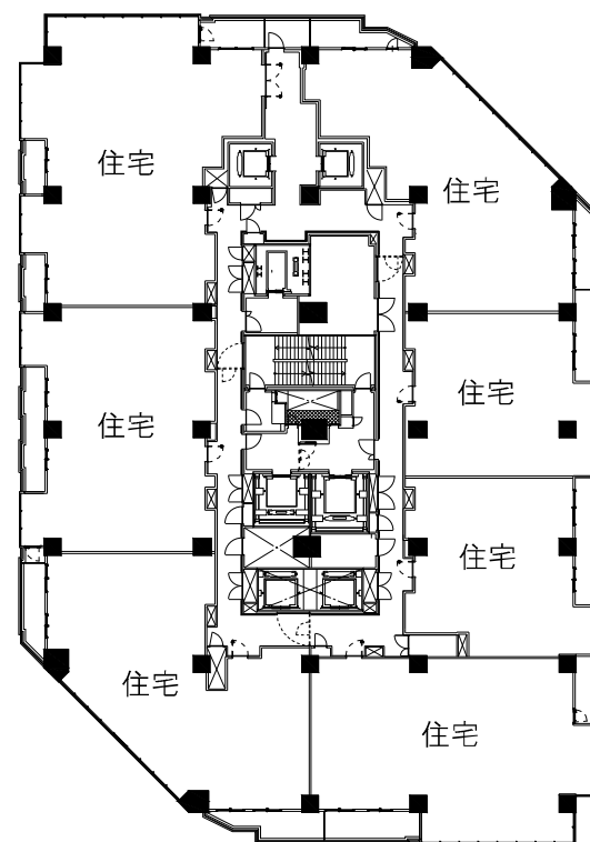
37~44階平面図 S=1/250(A1),S=1/500(A3)
