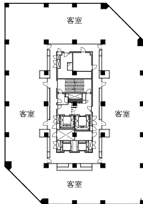
49階平面図 S=1/250(A1),S=1/500(A3)
