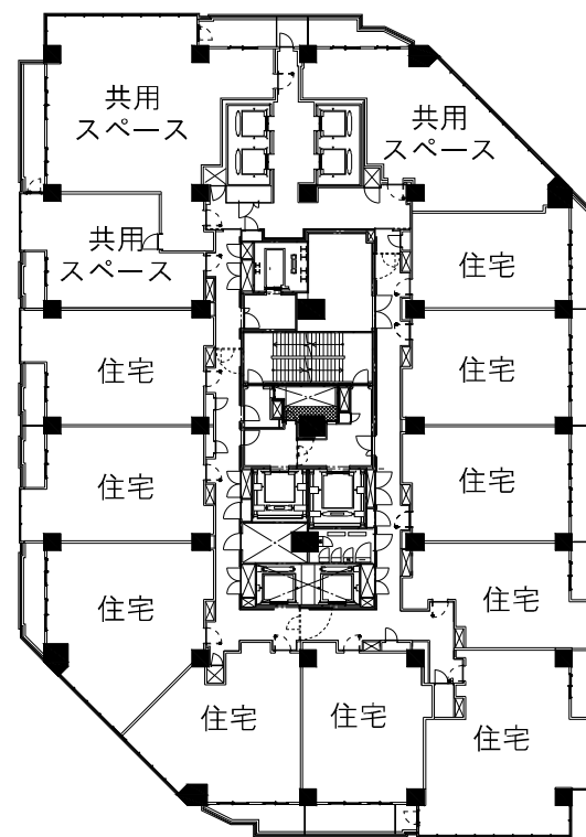
34階平面図 S=1/250(A1),S=1/500(A3)
