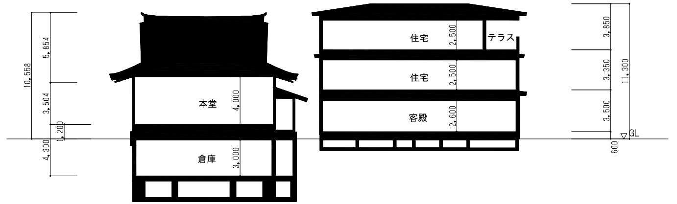
断面図 1
