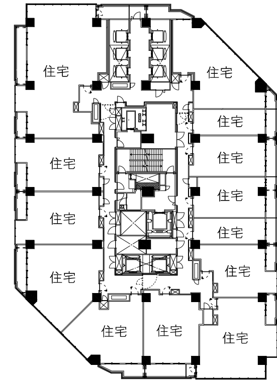
18階平面図 S=1/250(A1),S=1/500(A3)
