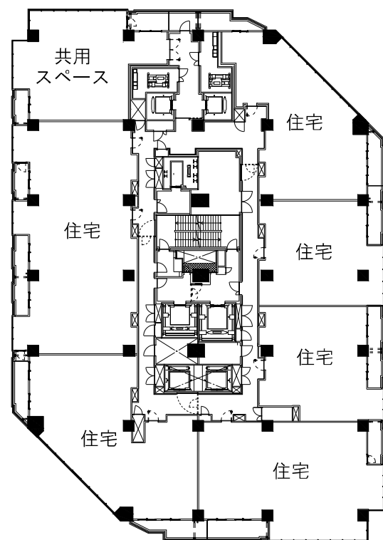
36階平面図 S=1/250(A1),S=1/500(A3)
