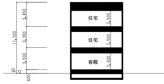
断面図 2
