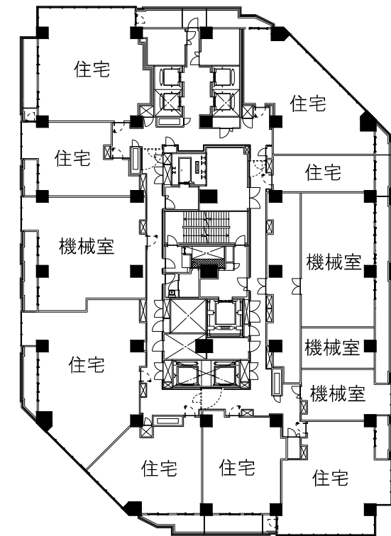
24階平面図 S=1/250(A1),S=1/500(A3)
