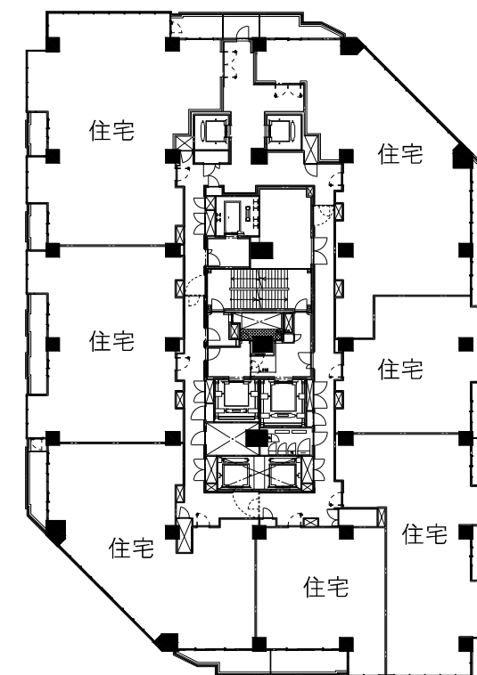
45階平面図 S=1/250(A1),S=1/500(A3)
