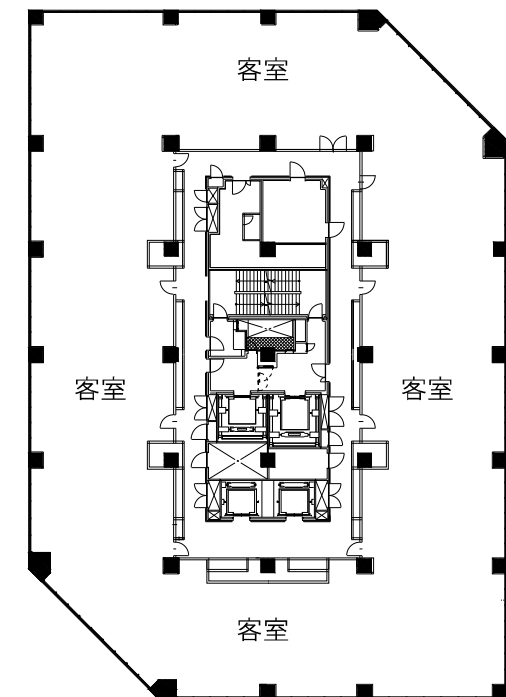
51階平面図 S=1/250(A1),S=1/500(A3)
