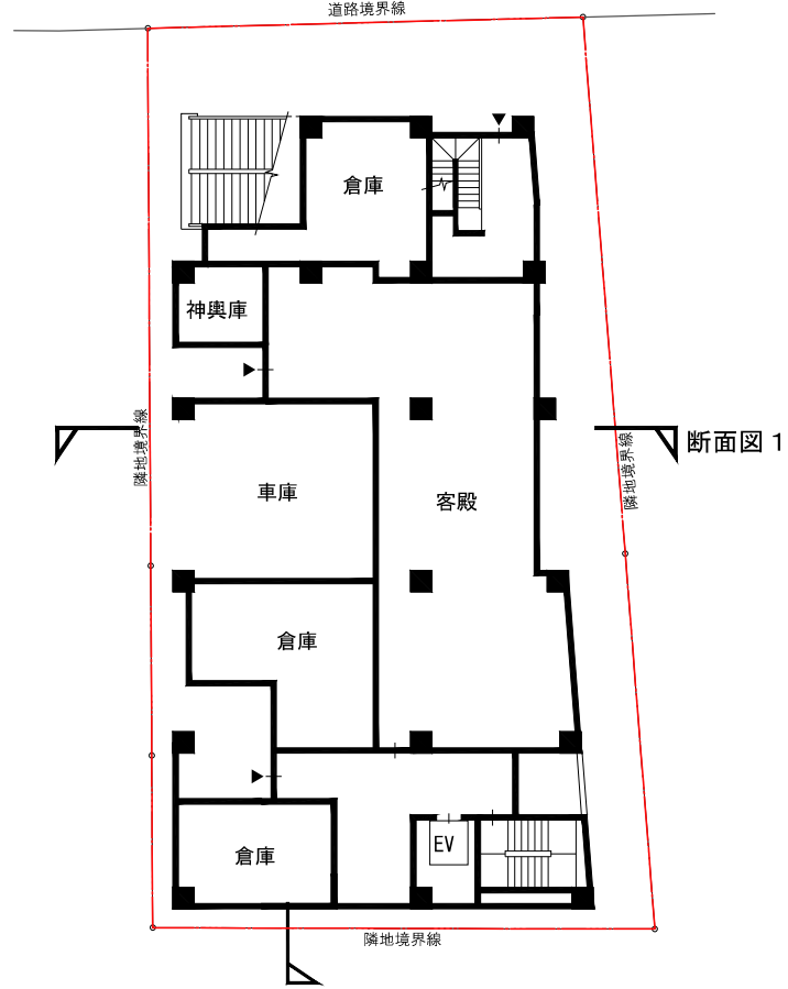
1階配置平面図
