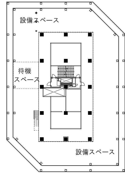
54階平面図 S=1/250(A1),S=1/500(A3)
