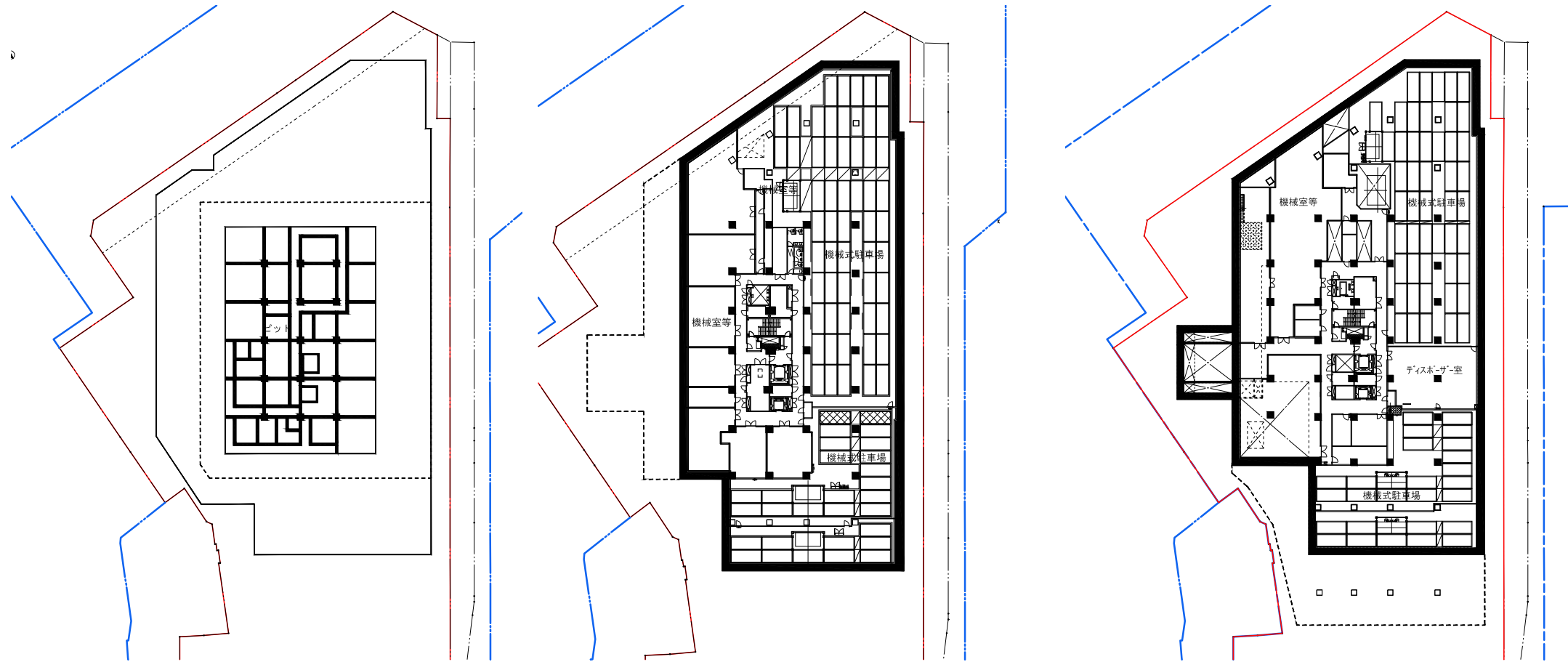
ピット階平面図 S=1/500(A1),S=1/1000(A3)
