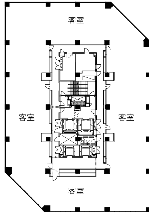
52階平面図 S=1/250(A1),S=1/500(A3)
