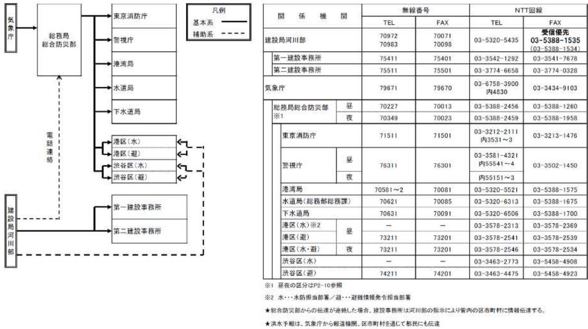
図3-5-4 渋谷川・古川洪水予報伝達系統図
