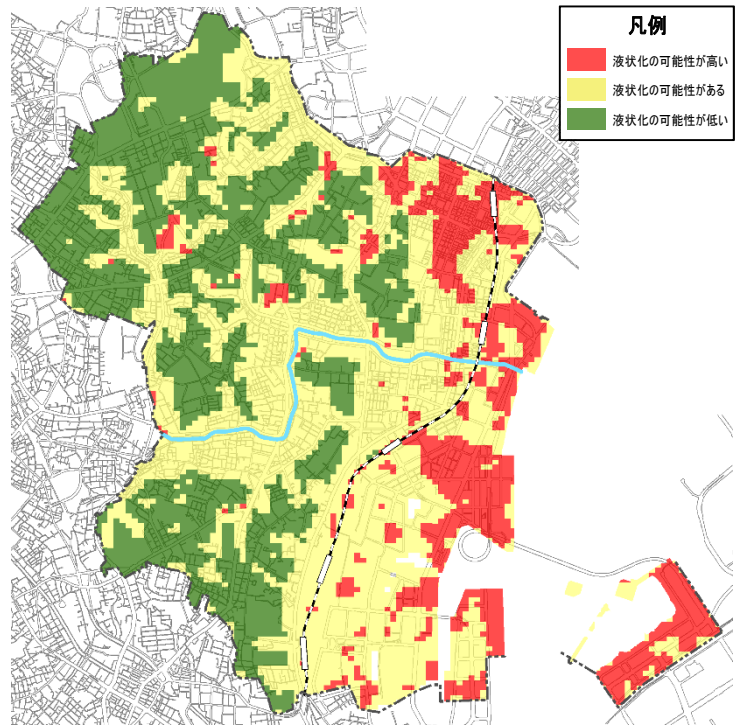
図1-2-15 液状化危険度分布
