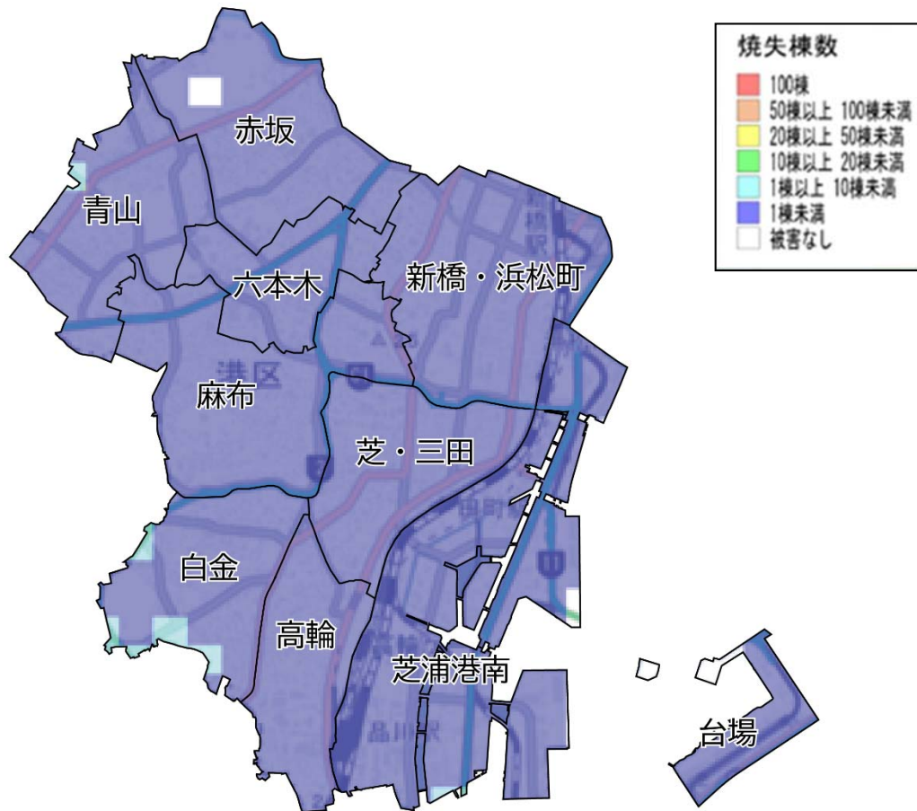
「東京都被害想定マップ」(令和4(2022)年)をもとに作成 図1-2-13 焼失棟数分布(都心南部直下地震(M7.3)冬夕方風速8m/s)
